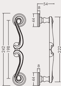
MANIGLIONE DIRITTO ROSETTE copriviti
