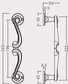
MANIGLIONE DIRITTO ROSETTE viti in vista
