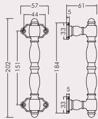
MANIGLIONE ZANCATO ROSETTE copriviti
